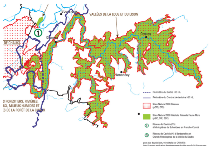
Figure 1 : Vallée de la Loue et du Lison – Sites Natura 2000
